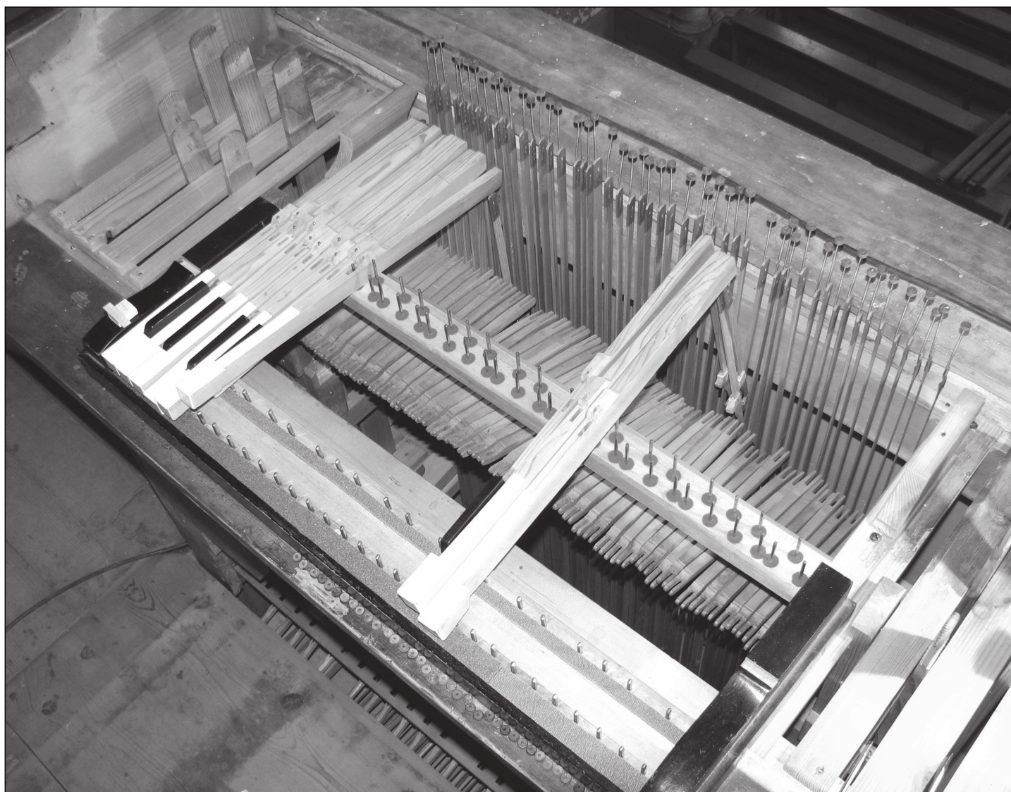
Manuálové klaviatury při montáži po opravě.
