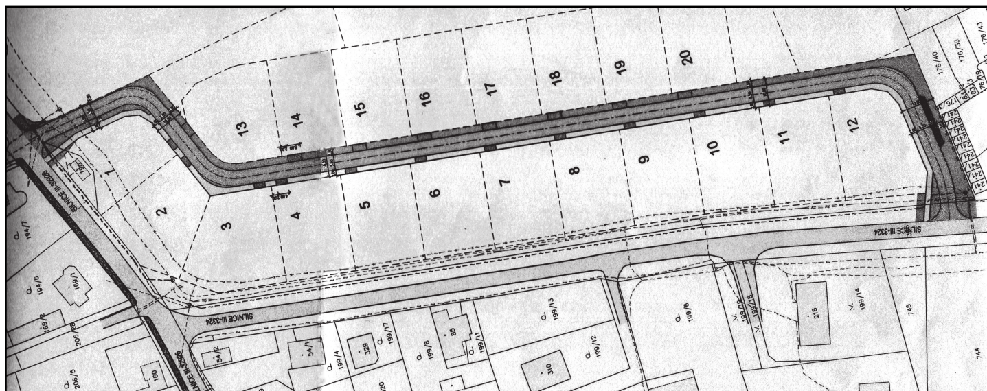
Rozparcelování pozemku a komunikace viz výkresová dokumentace.
